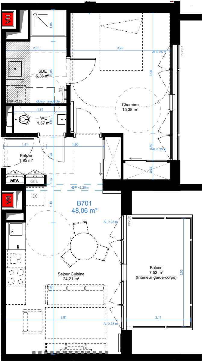
Plan appartement B 701 - 1 : 75
