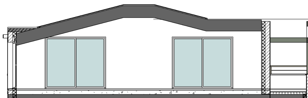
Coupe sur séjour 1206
