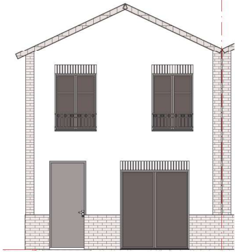
FAÇADE SUD
