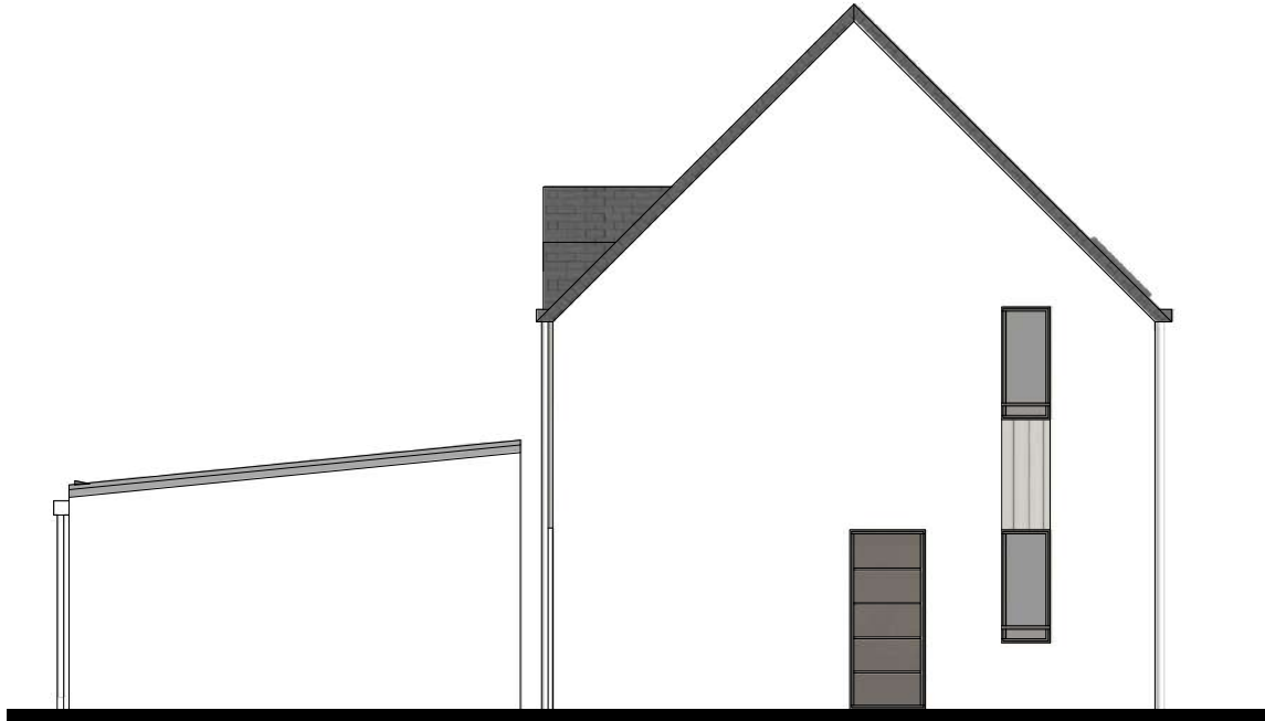
Pignon AVANT
