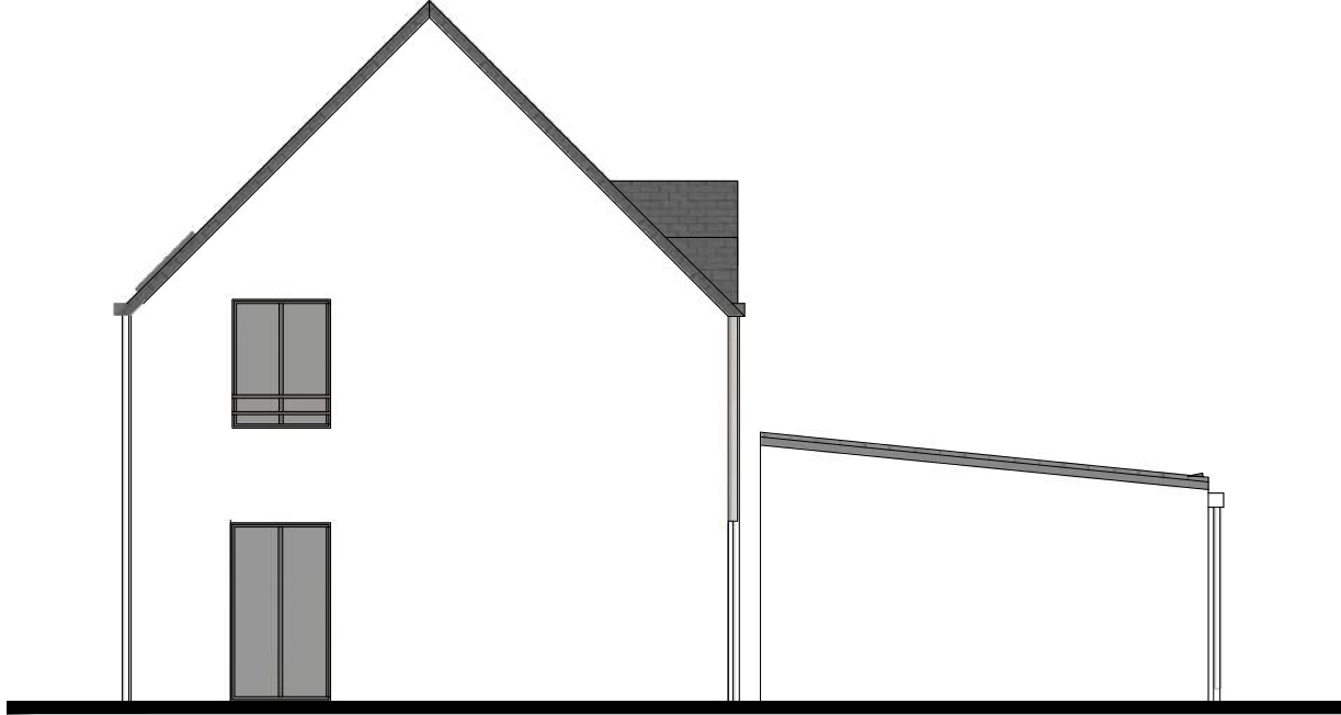
Pignon AVANT
