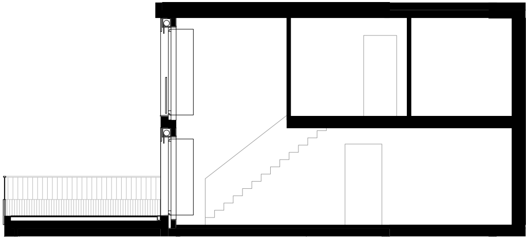
c Coupe du logement duplex
