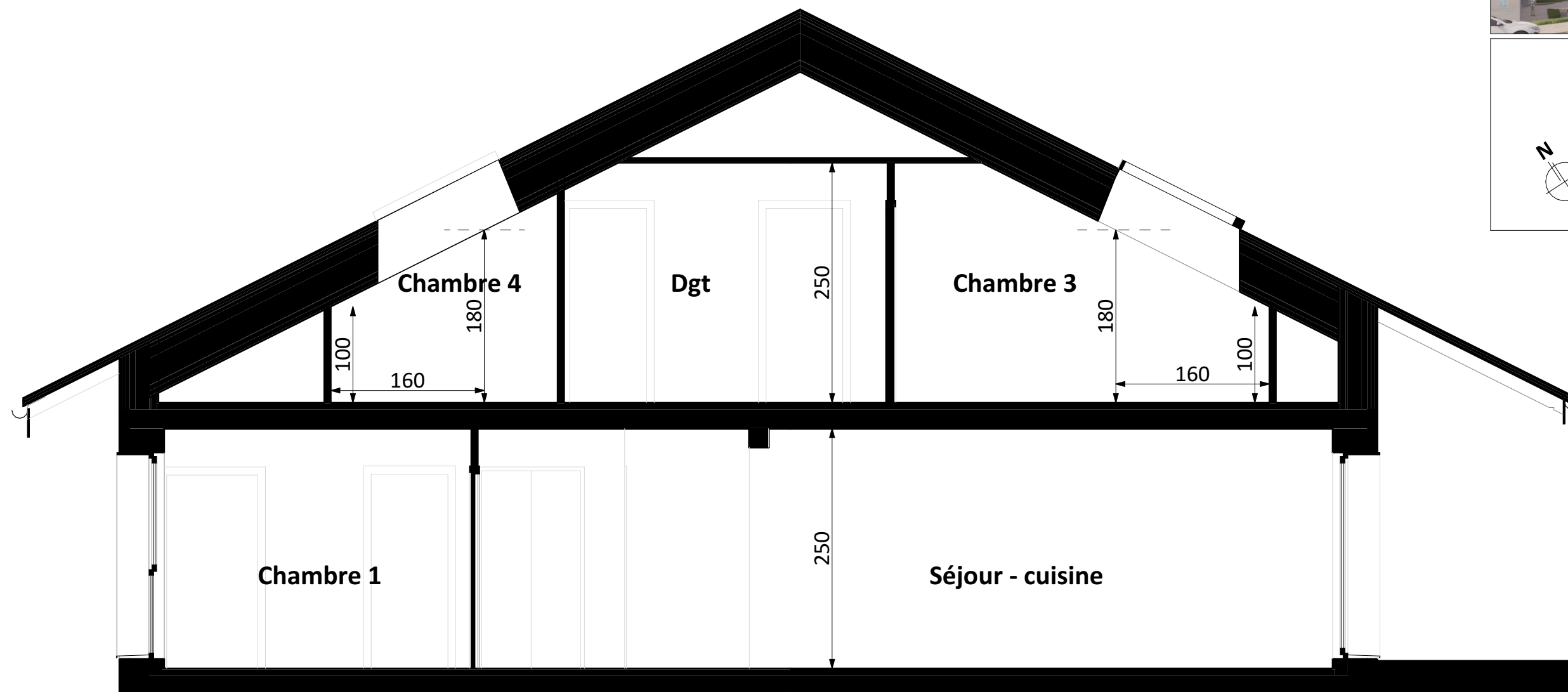
Coupe 1
