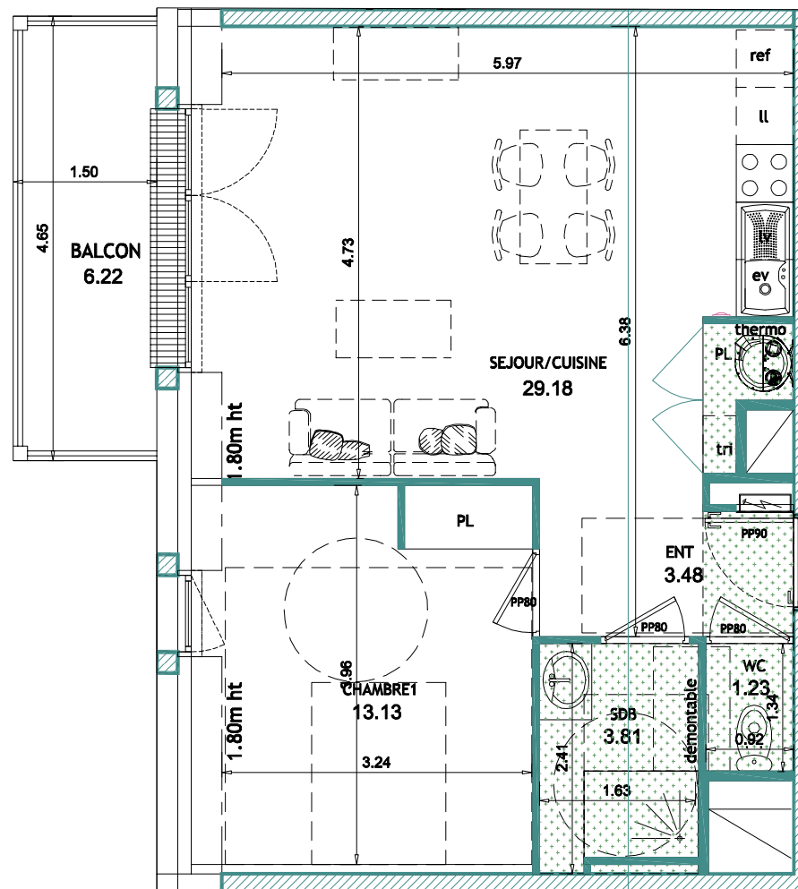
Plan de vente LA 306-ech 1/50ème
